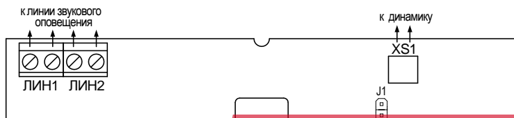
Рис.1 Плата «АС-2-2». Схема соединений
